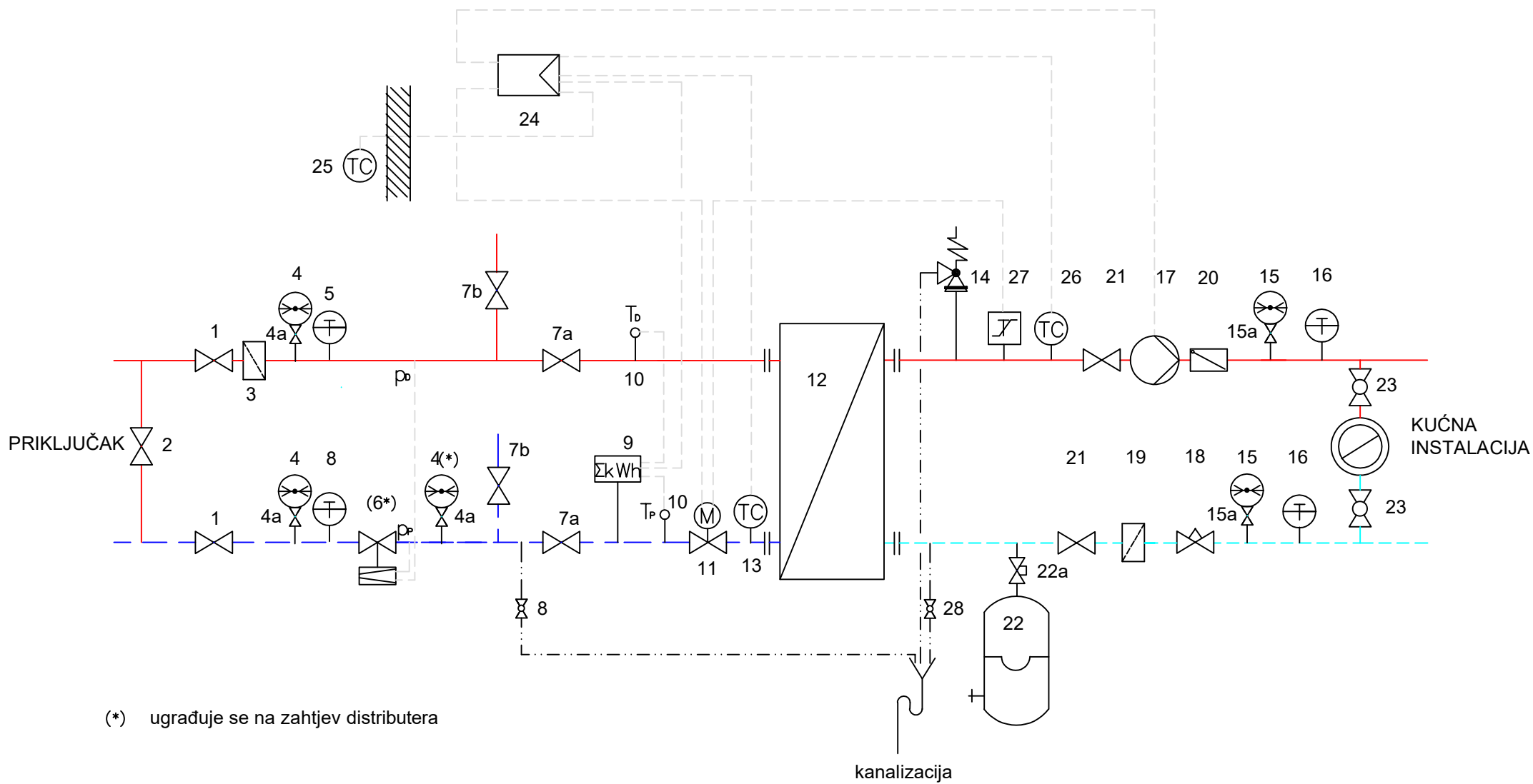
PRILOG 2: TEHN. ŠEMA INDIREKTNE TOPLOTNE PREDAJNE STANICE
